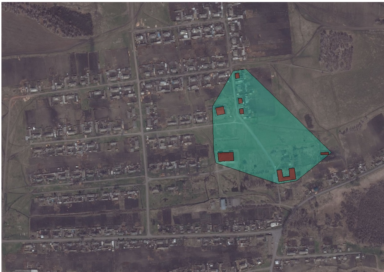
Рисунок 1.2 – Существующая зона действия источника тепловой энергии села Семенниково
