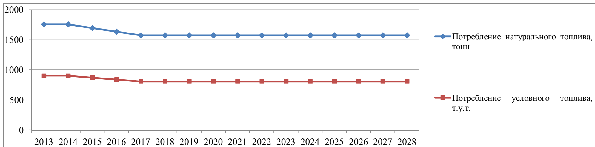
Рисунок 8.1. Перспективный топливный баланс котельной с. Нижний Суэтук
