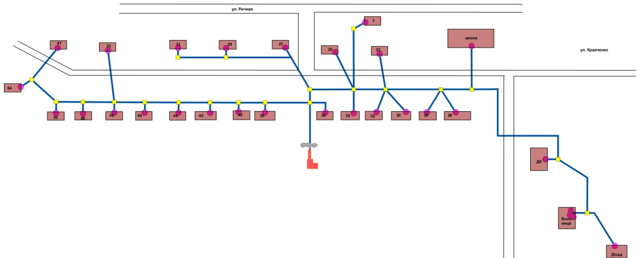
Схема тепловых сетей от котельной пос. Ойский
