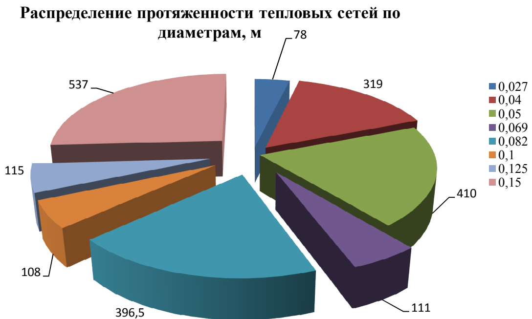
Рисунок 1.5. Распределение тепловых сетей по диаметрам участков
