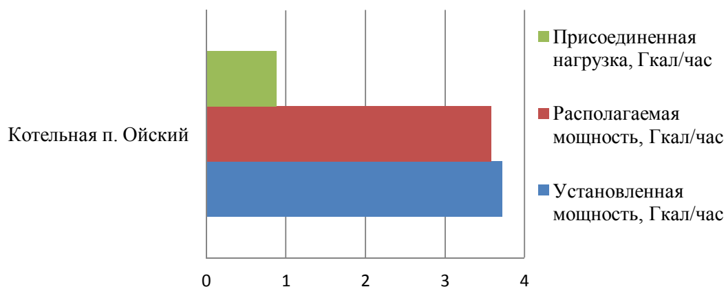
Установленная, располагаемая мощность источников тепловой энергии, присоединенная нагрузка, Гкал/час
