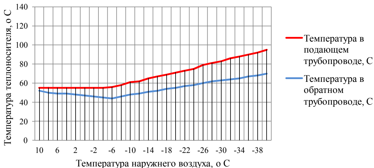
Рисунок 1.3 Температурный график работы системы теплоснабжения
